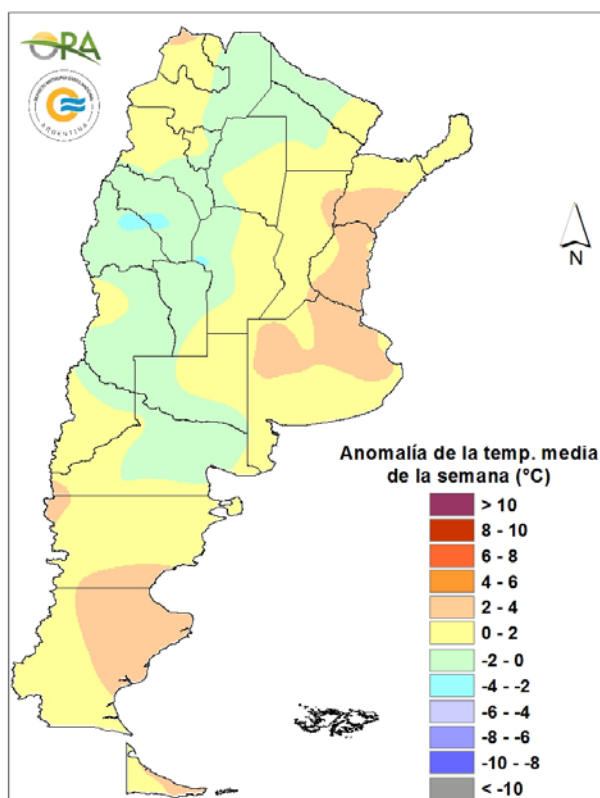
Anomalía de la temperatura media de la semana del 18/03/2025 al 25/03/2025
