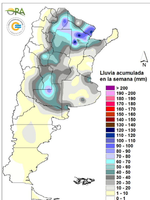
Precipitaciones acumuladas en la semana del 18/03/2025 al 25/03/2025
